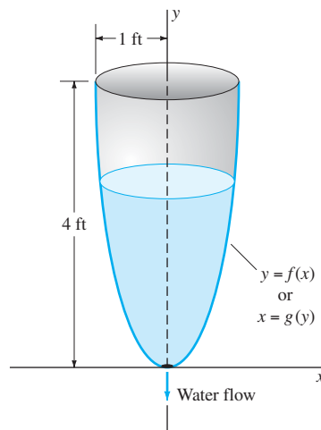
FIGURE 1.4.10. The clepsydra.
